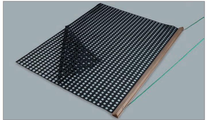
Holz-Schleppnetz Spezial doppelt Mit doppeltem Spezial-PVC-Gewebe, Holzschiene und Zugseil. Arbeitsbreite 200 cm. Netztiefe 150 cm. Nr. 41041
