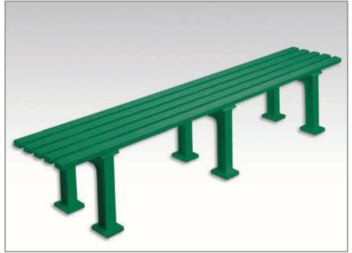
Bank Stuttgart 200 cm Länge, grün 3 Vollkunststoff-Füße sowie 5 Mehrkammerprofil-Latten, ohne Lehne daher beidseitig verwendbar, hoher Sitzkomfort. Gewicht ca. 12 kg. Nr. 412213 grün Stück € 144,00
