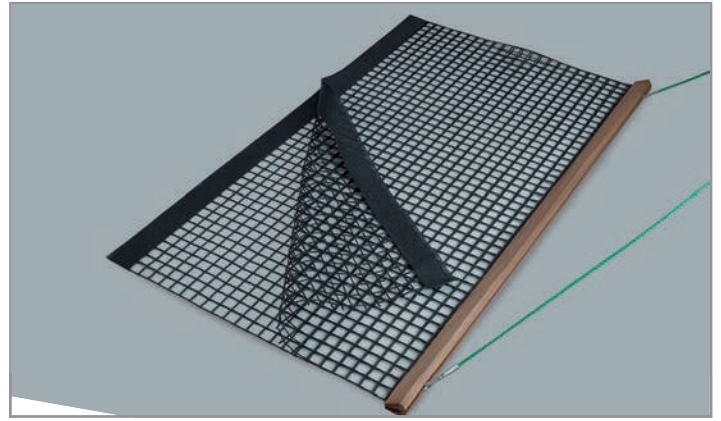
Holz-Schleppnetz PVC doppelt Mit Holzschiene, Zugseil und doppelt PVC-beschichtetem Netz. Arbeitsbreite 200 cm. Netztiefe 115 cm. Nr. 41020
